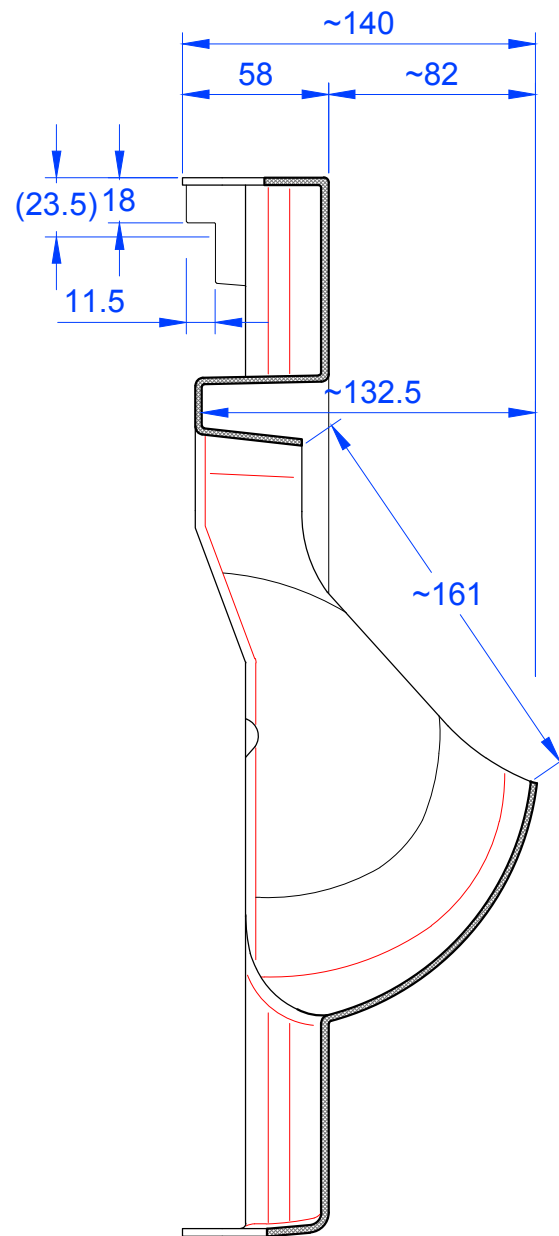
Schnitt B-B
