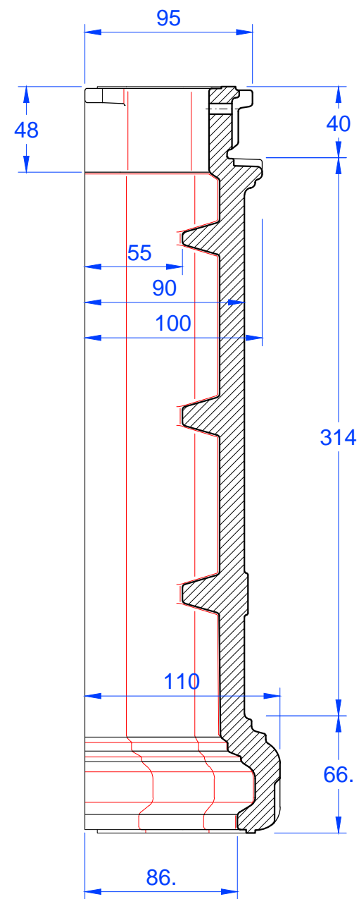
Schnitt A-A
