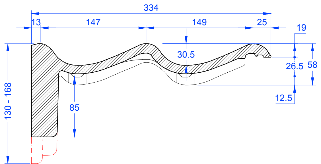
Schnitt A-A
